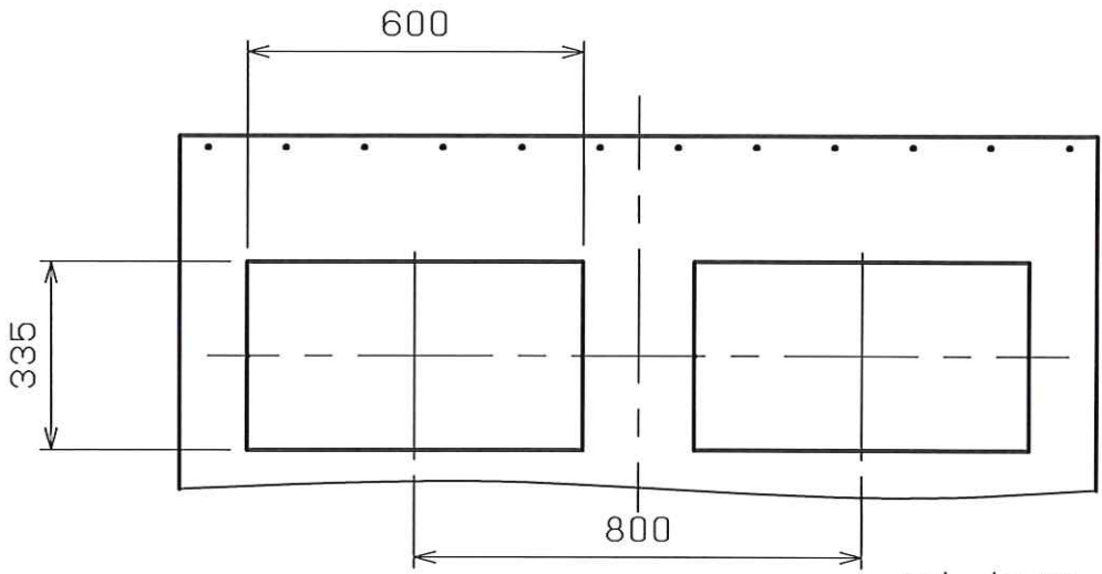
D矢视图
