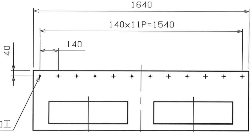
① 詳細図
