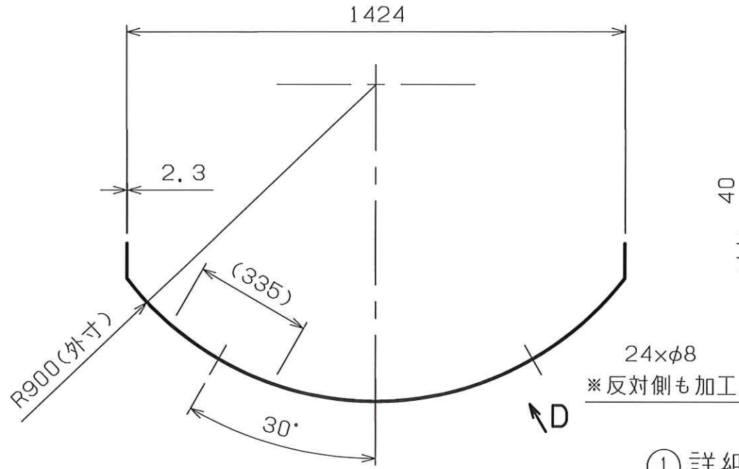
① 詳細図
