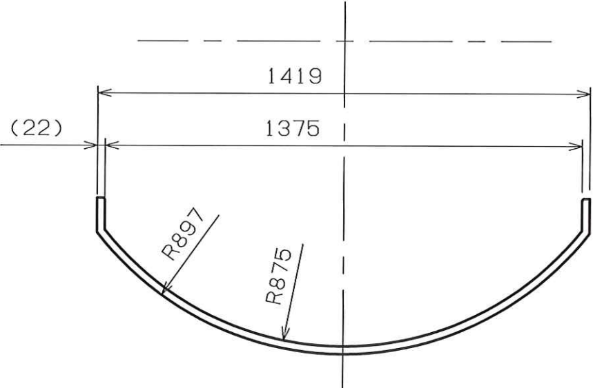
⑤ 詳細図
