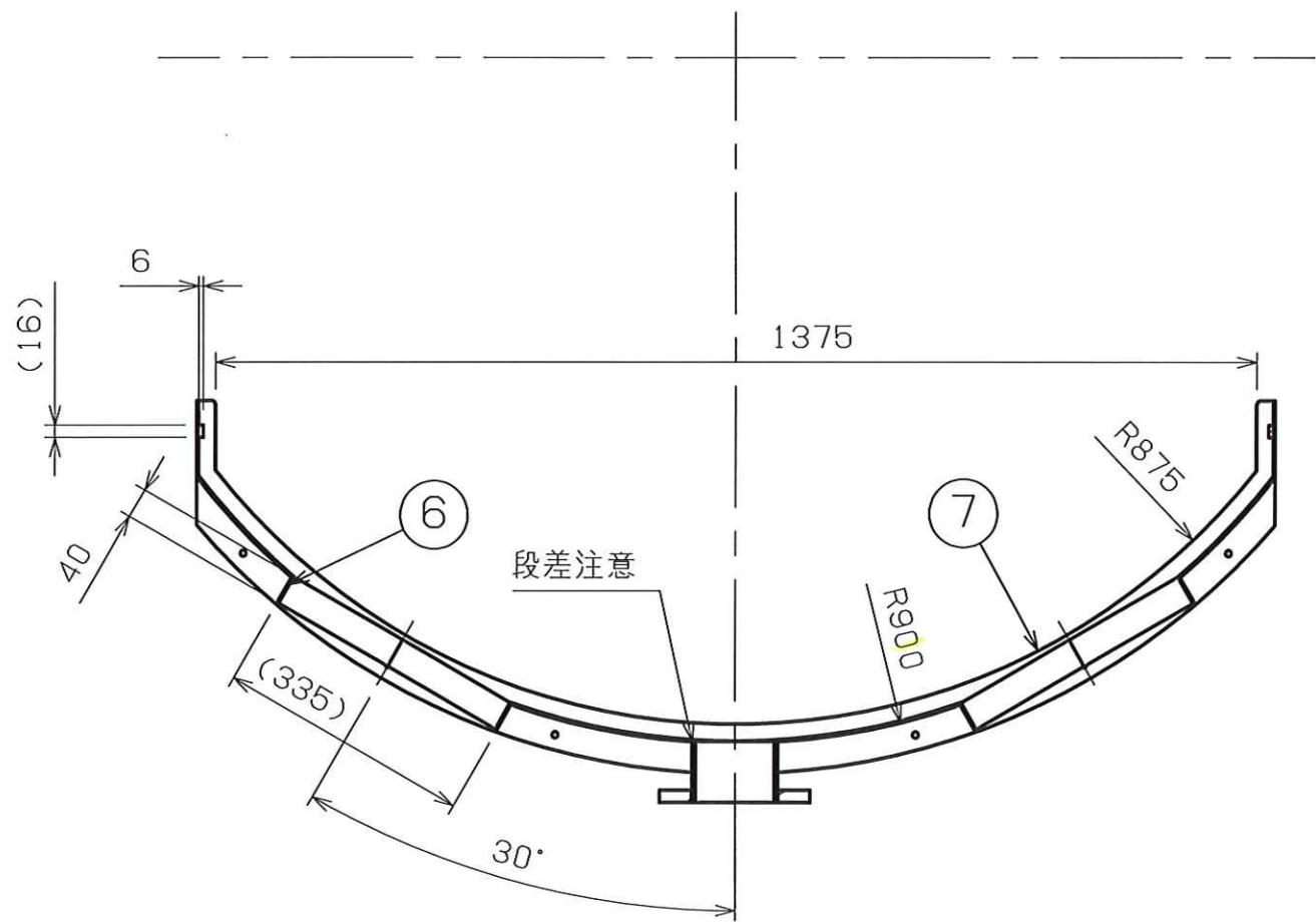
B-B断面図
